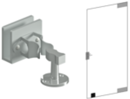
1873 Conj. Fixador de Porta para Piso (Recorte)
